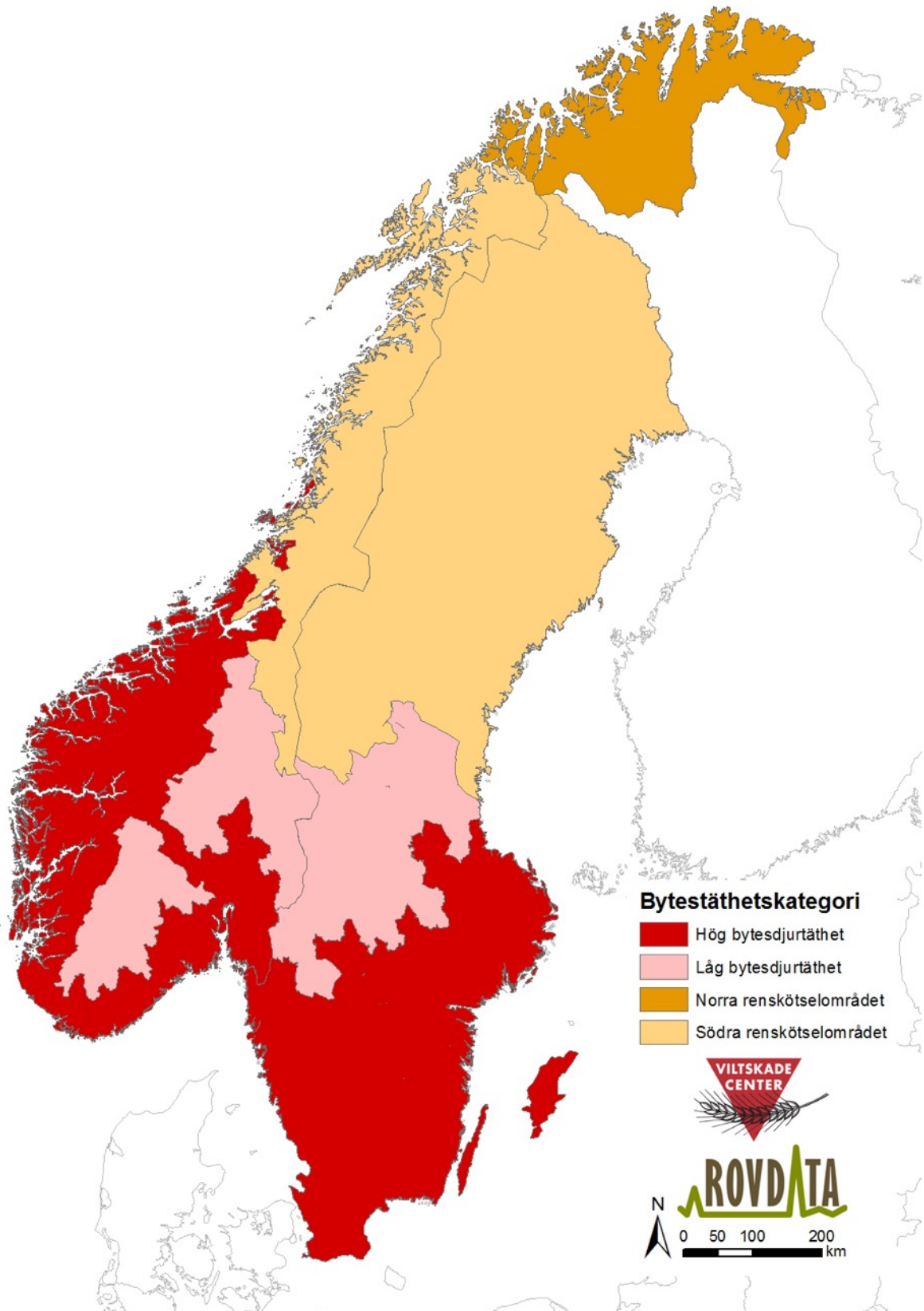
Figur 1. Avståndskriterierna och omräkningsfaktorer som används varierar med tätheten av stora bytesdjur (Gervasi mfl. 2013). Skandinavien är indelat i fyra kategorier: 1- norra renskötseområdet, 2- södra renskötseområdet, 3- områden med «låg» bytesdjurstäthet, och 4- områden med «hög» bytesdjurstäthet.
