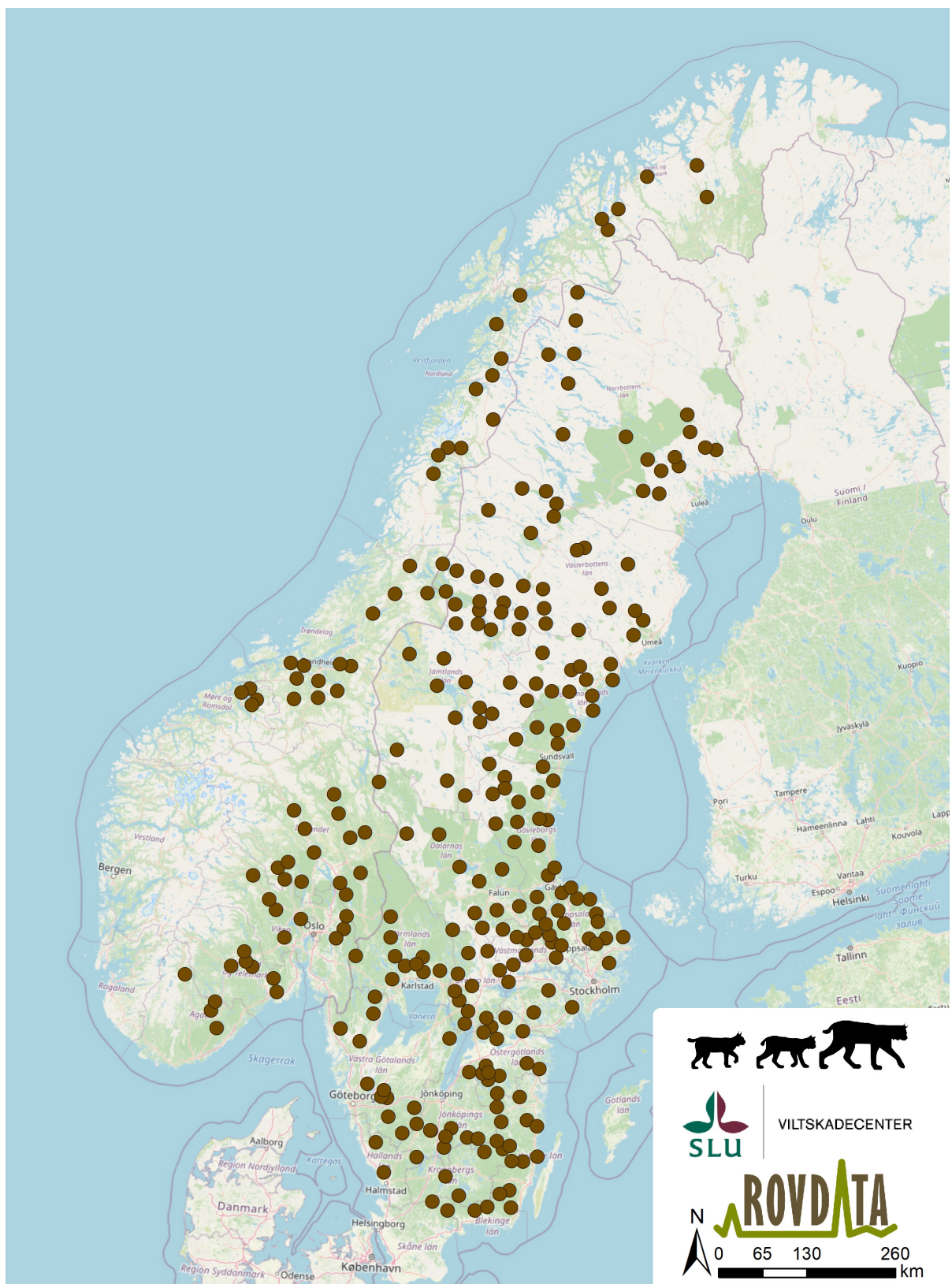
Figur 2. Kartan visar funna familjegrunder i Skandinavien under säsongen 2020/2021. Källa: Rovbase.
